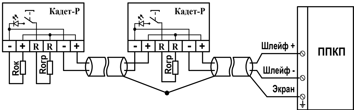
Рис. 3 Схема подключения извещателей с нормально-разомкнутым контактом к ППКП с постоянно-токовым питанием ШПС (с увеличением тока в режиме «ПОЖАР»)
