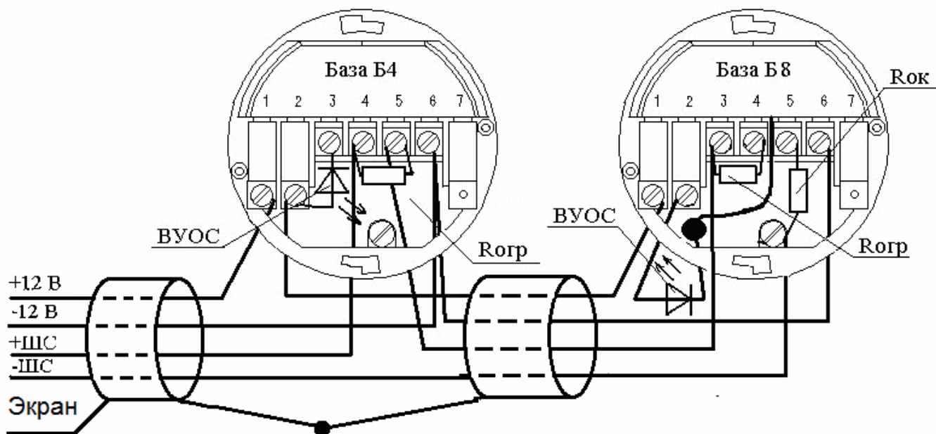
Схема подключения извещателей к пожарным ППКП посредством баз Б4 и оконечной базы Б8
